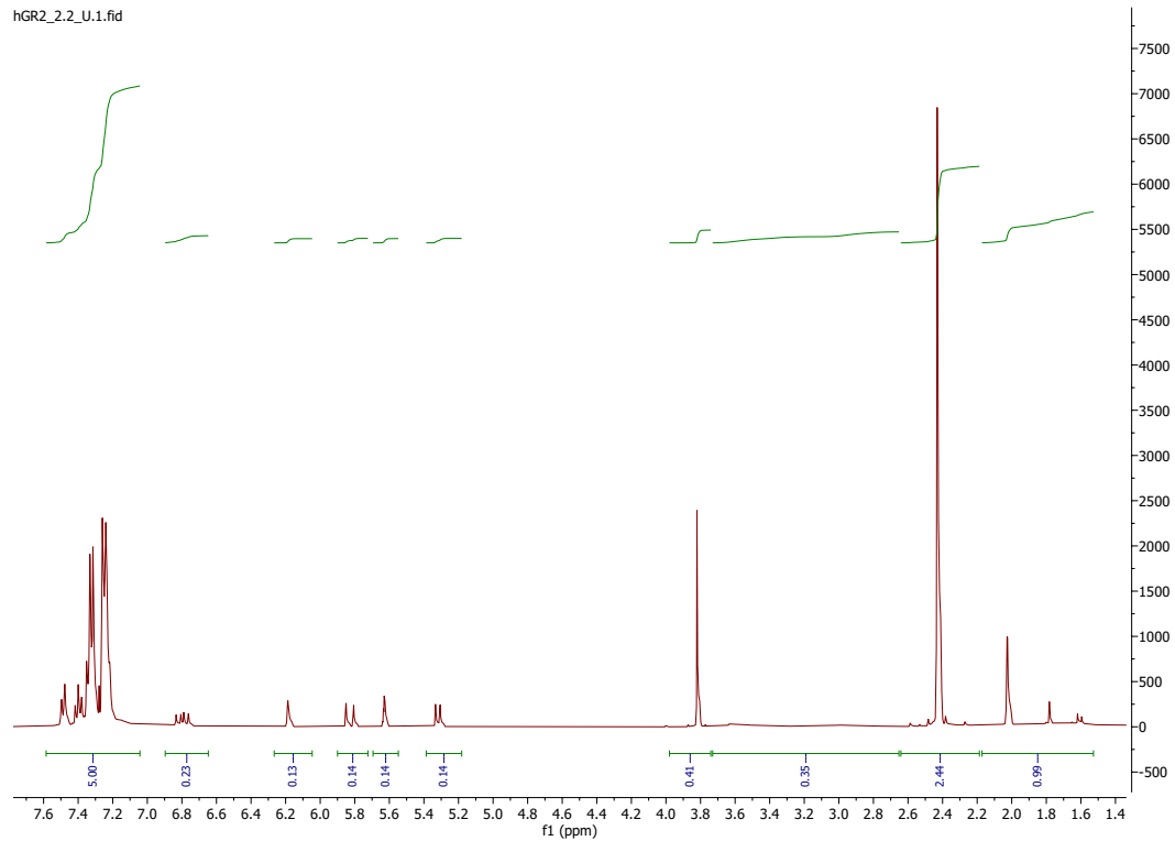
Abb. 16: NMR-Spektrum der Polystyrol- co -Polymethylmethacrylatprobe vor der Fallung.
